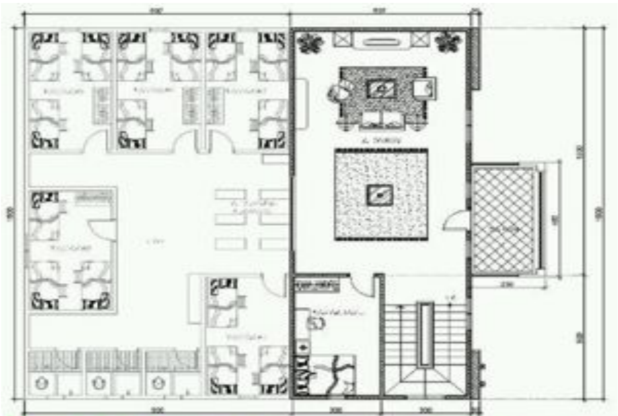
DENAH LANTAI 2 (dua)
